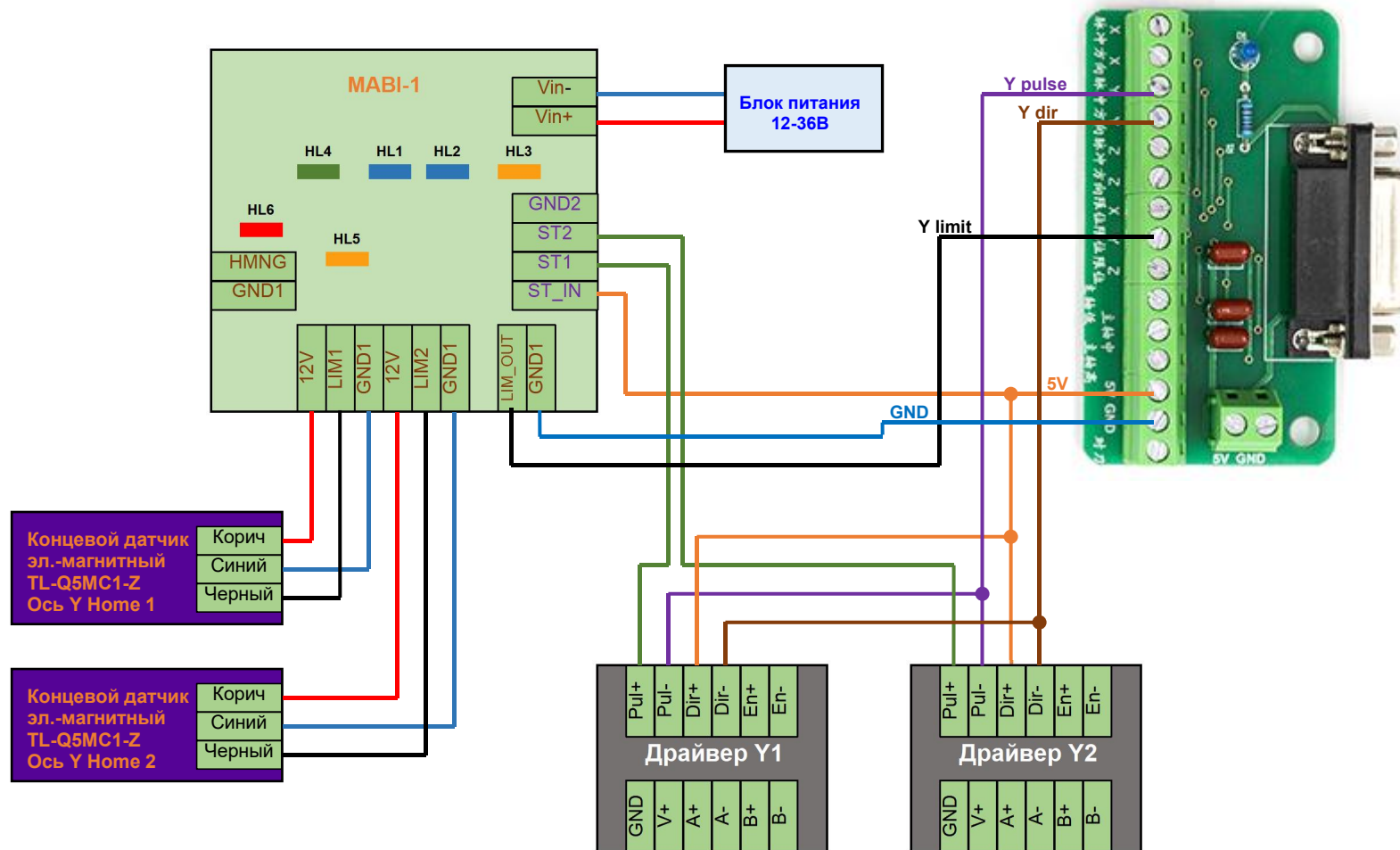
Схема подключения платы выравнивания портала MABI-1 к плате развязки NC Studio 5 (схема с подключением драйверов по общему плюсу)
