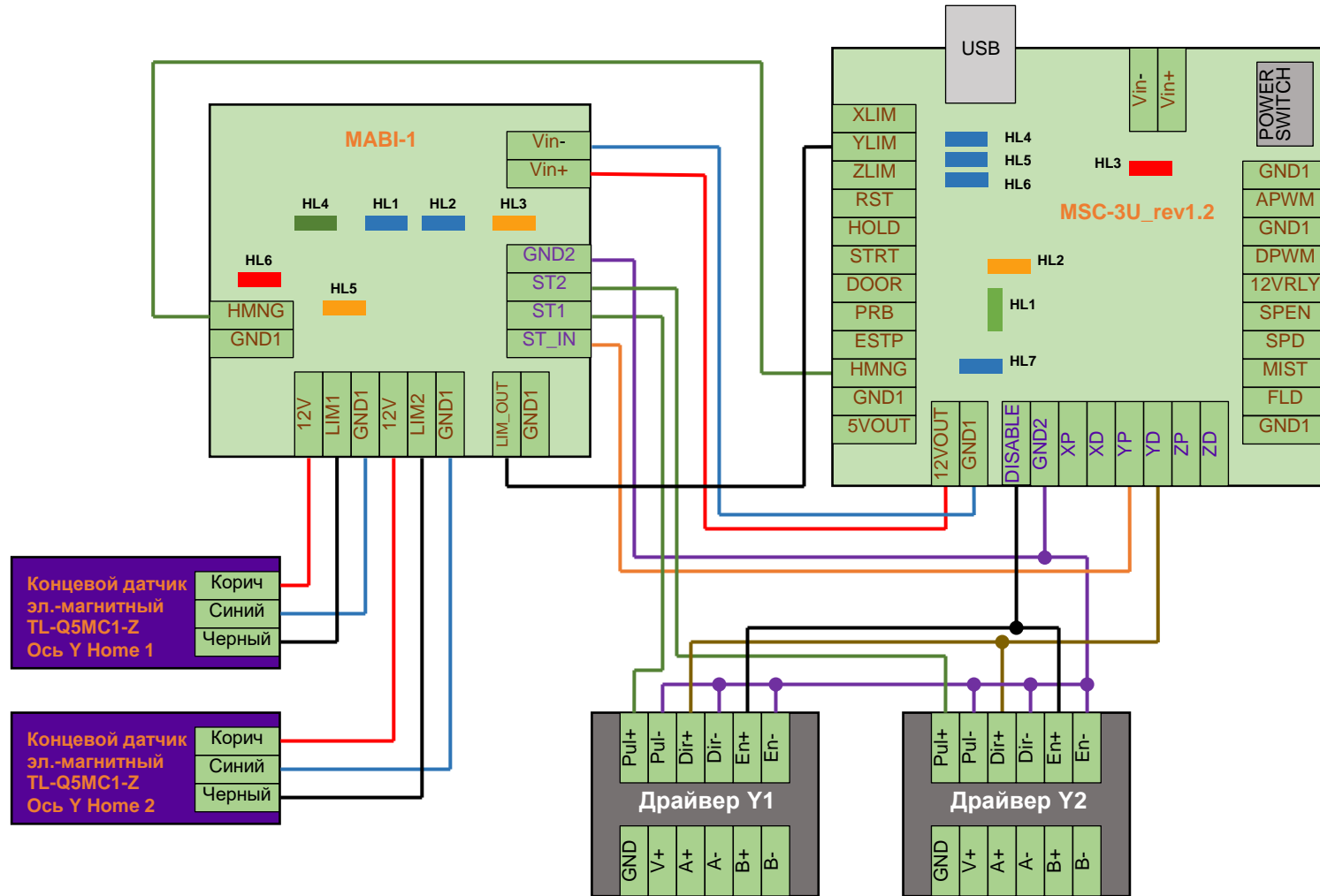
Схема подключения платы выравнивания портала MABI-1 к ЧПУ-контроллеру MSC-3U
